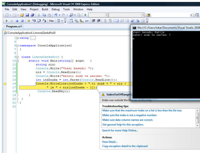
Slika 22: Pri delovanju programa je prišlo do izjeme IndexOutOfBounds Vir: Lasten
