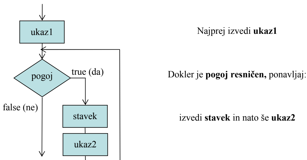
Slika 19: Diagram poteka za for zanko Vir: Lasten
