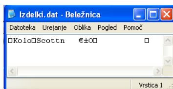
Slika 35: Binarna datoteka odprta z beležnico Vir: Lasten
